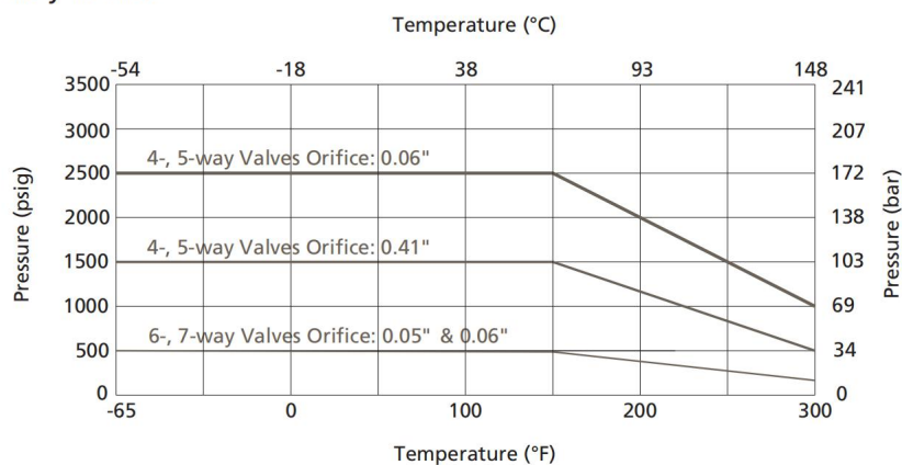
4-, 5-, 6-, 7-way Valves
