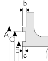
Type D Groove face
